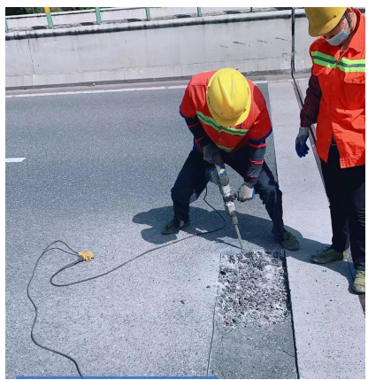
巴陕段巴陕向 809 处路面坑洞修补
