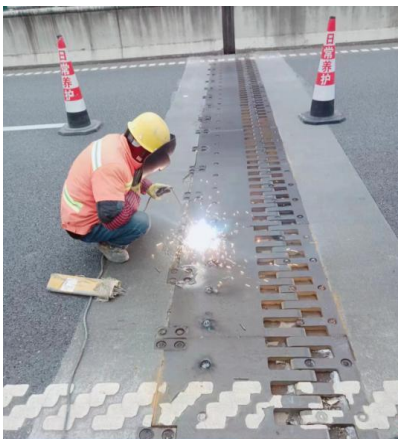
巴陕段陕巴向 812+080 处焊接桥梁伸缩缝梳齿板
